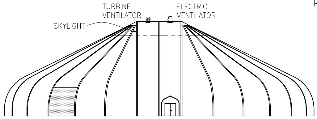
ELEVATION 1:400
