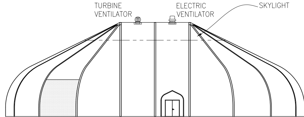
ELEVATION 1:300
