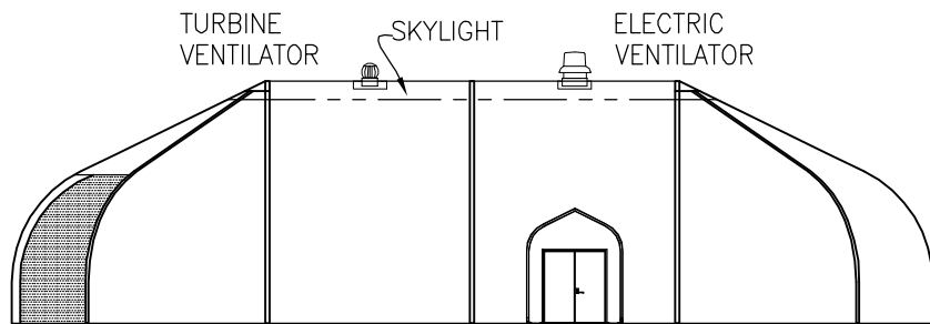
ELEVATION 1:250
